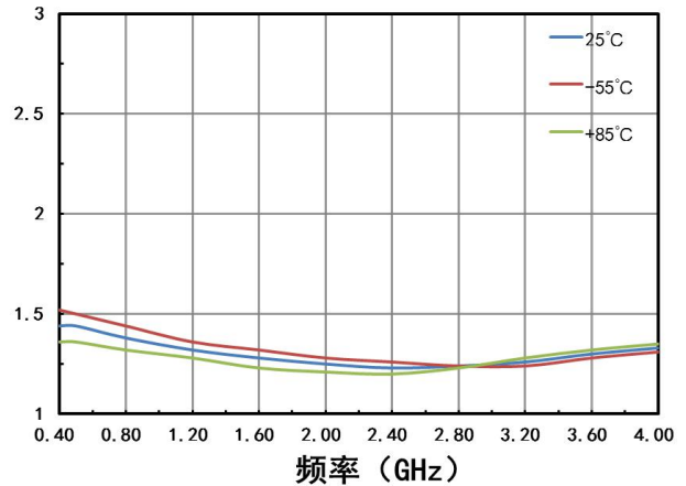
输出驻波比 VS 温度
