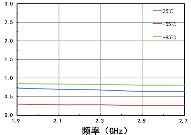
噪声系数 (dB) VS 温度
