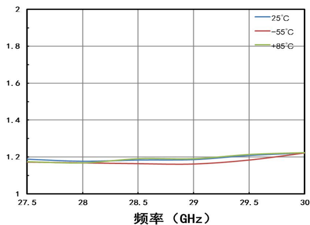
输出驻波比
