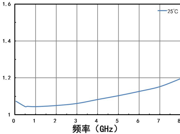
开态输入驻波
