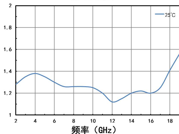
输出驻波比
