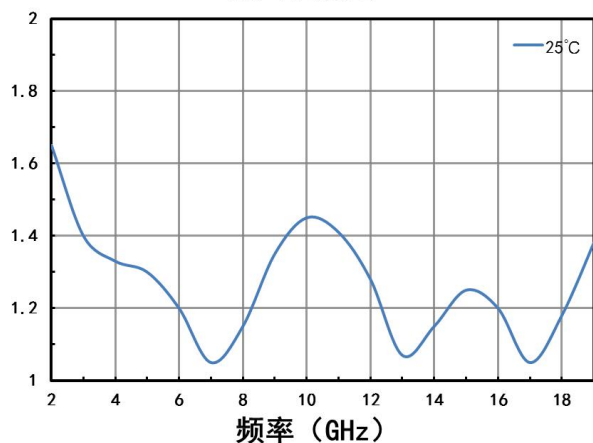
输入驻波比
