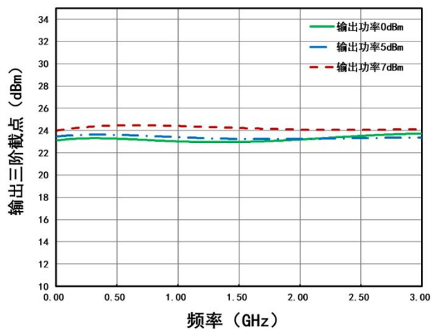
典型测试曲线: (50Ω系统, V_{dd}=+5V , I_{dd}=25mA )
