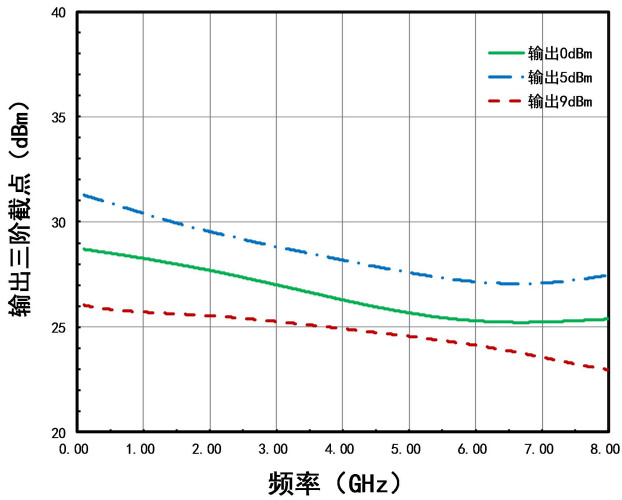
典型测试曲线 2: (50Ω系统, V_{dd}=+5V , I_{dd}=62mA )
