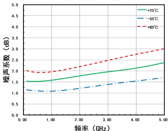
噪声系数VS. 温度
