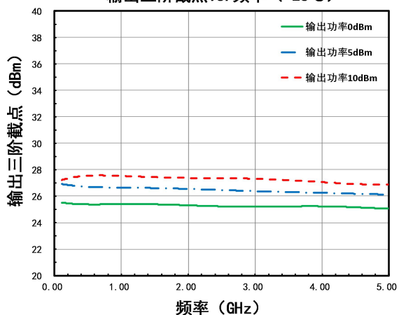
输出三阶截点VS. 频率 (+25°C)
