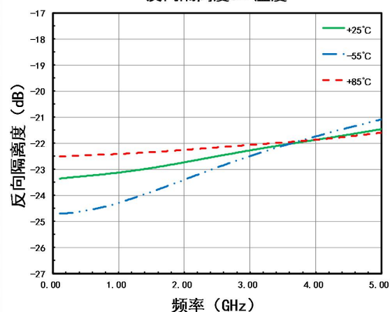
反向隔离度VS. 温度
