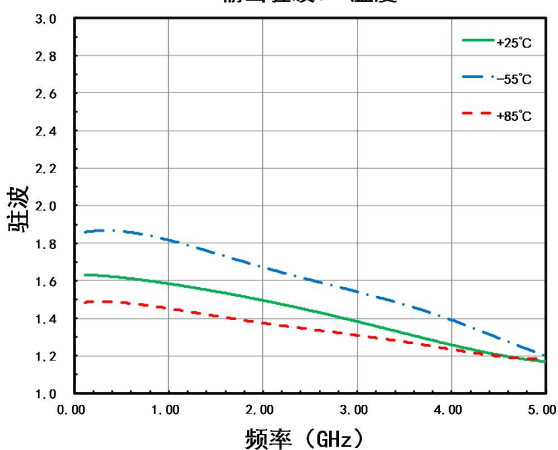
输出驻波VS. 温度
