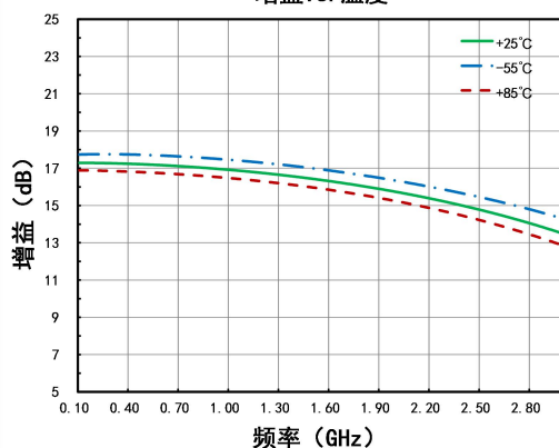
增益VS. 温度
