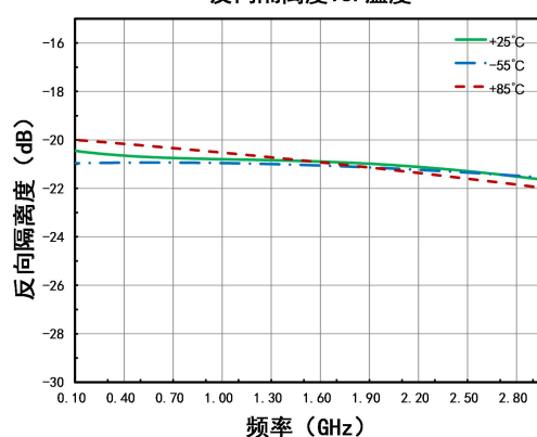
反向隔离度VS. 温度
