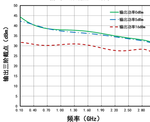
输出三阶截点VS. 频率(+25℃)
