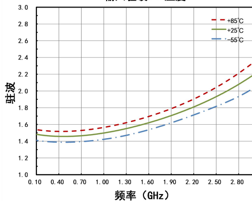
输入驻波VS. 温度
