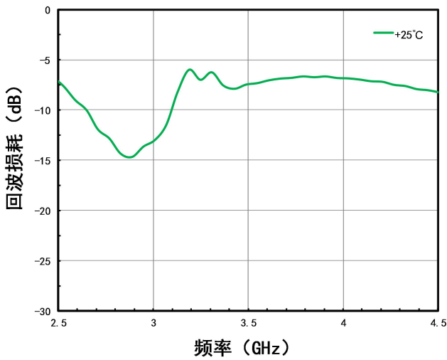
回波损耗VS. 温度
