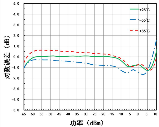
对数误差 VS. 温度 4GHz
