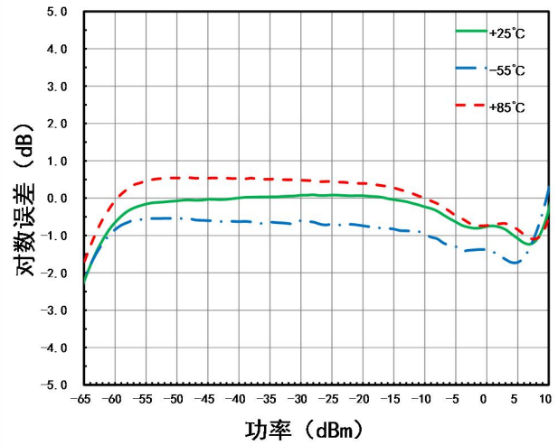
对数误差 VS. 温度 2GHz
