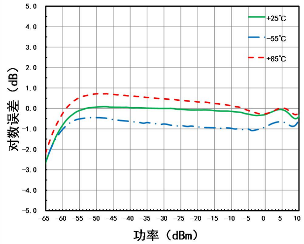
对数误差 VS. 温度 1GHz
