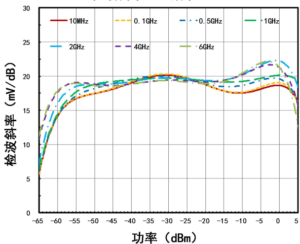
检波斜率 VS. 频率 (+25°C)
