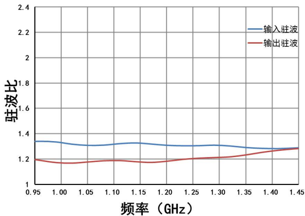
频率VS驻波比@V T =0V
