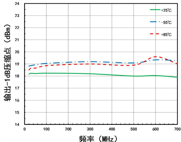
输出-1dBm压缩点VS. 温度
