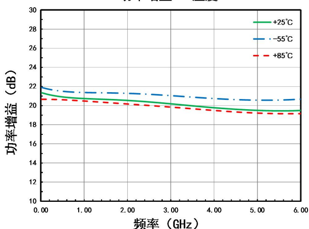
功率增益VS. 温度
