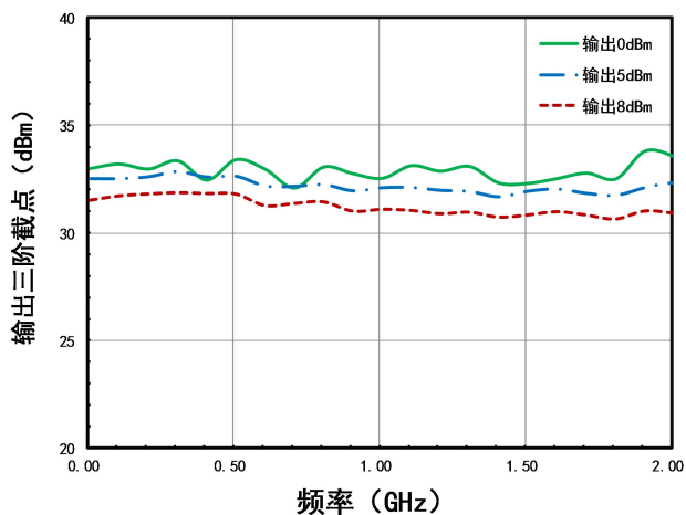
输出三阶截点VS. 频率(+25℃)
