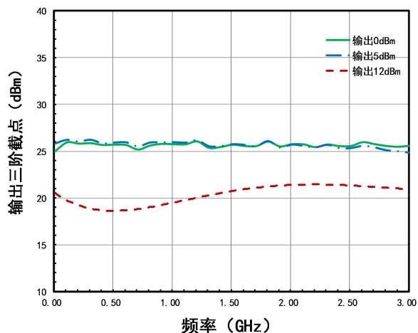
典型测试曲线: (50Ω系统, V_{dd}=+5V , I_{dd}=42mA )
