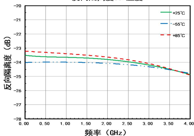
反向隔离度VS. 温度
