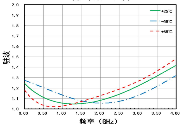
输入驻波VS. 温度
