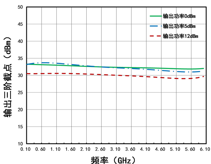
输出三阶截点VS. 频率(+25°C)
