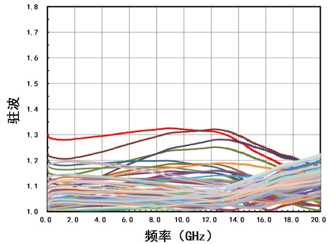
输入驻波 VS. 全部衰减态 25°C
