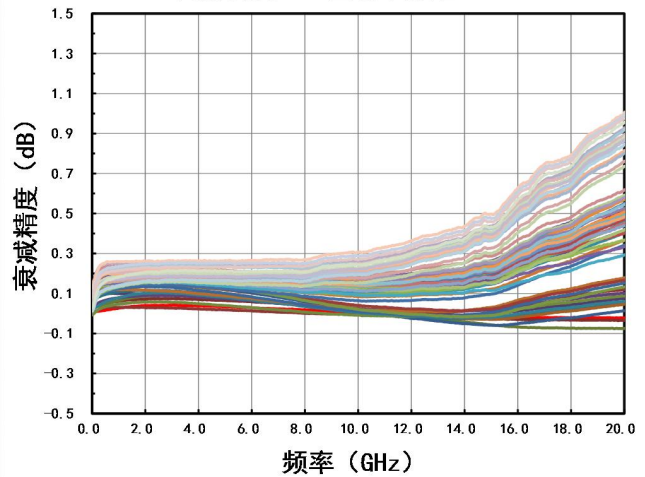
衰减精度 VS. 全部衰减态 25°C
