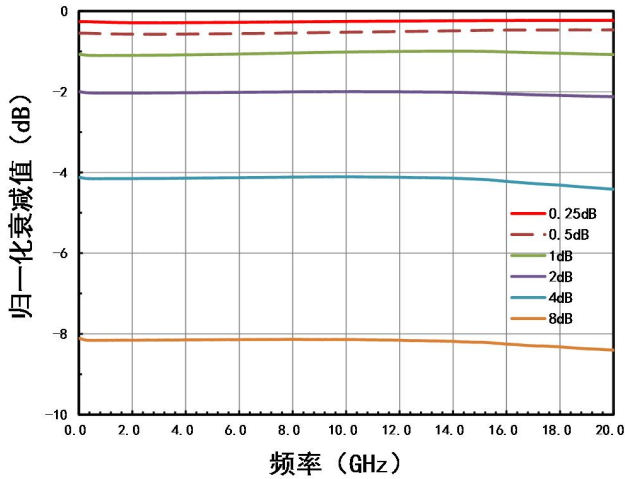
归一化衰减值 VS. 基本衰减态 25°C
