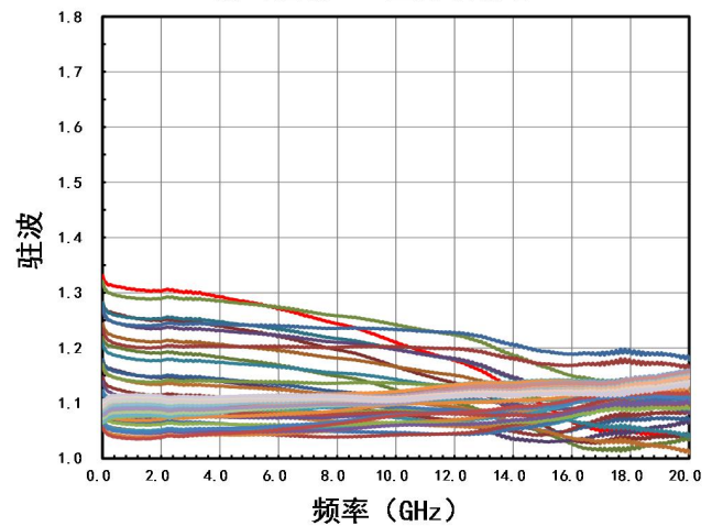
输出驻波 VS. 全部衰减态 25°C
