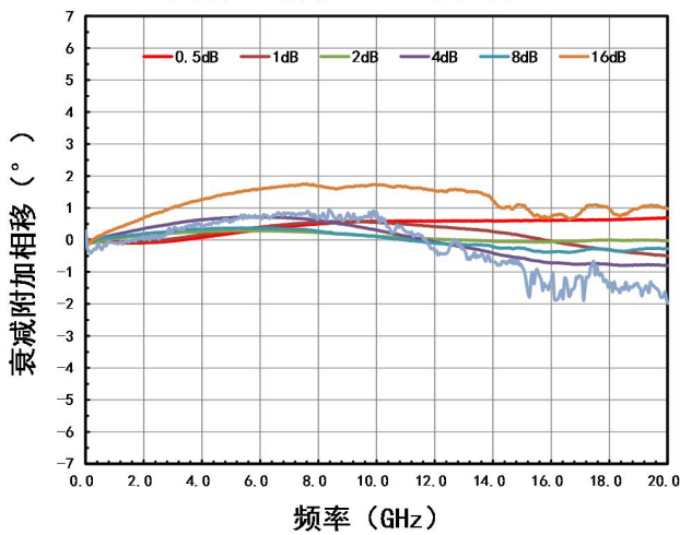
衰减附加相移 VS. 基本衰减态 25°C
