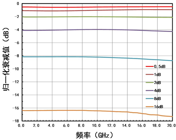
归一化衰减值 VS. 基本衰减态 25°C
