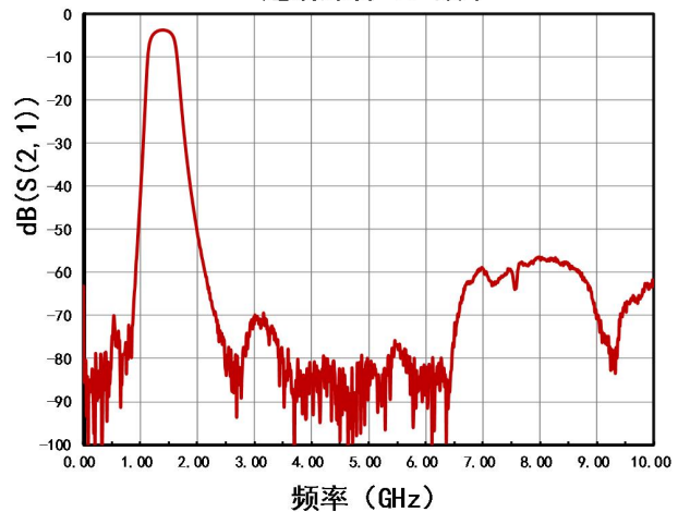
远端抑制 VS 频率
