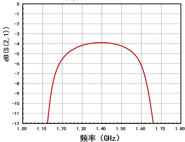
通带插损 VS 频率
