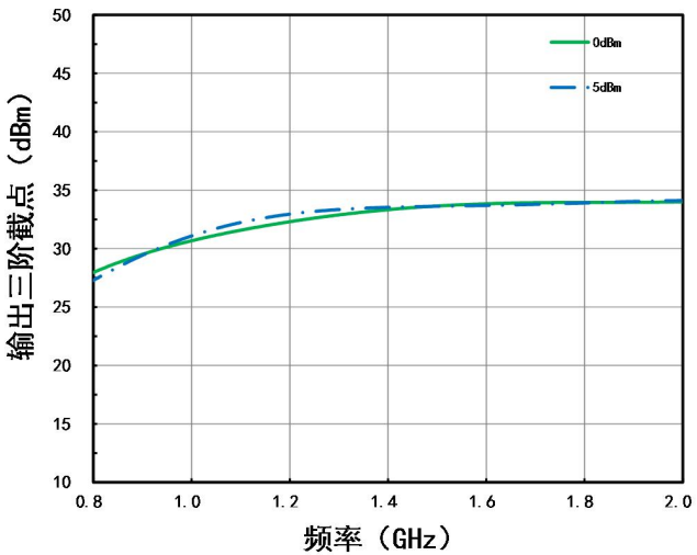
输出三阶截点VS. 频率
