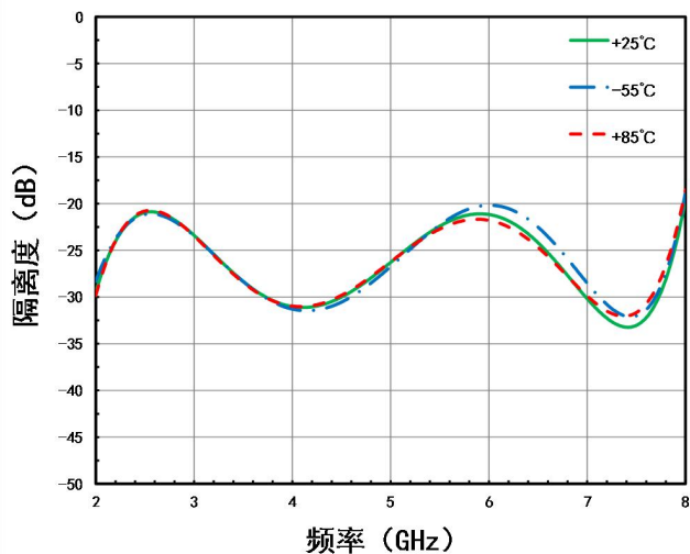
RF1-RF2隔离度 VS. 温度
