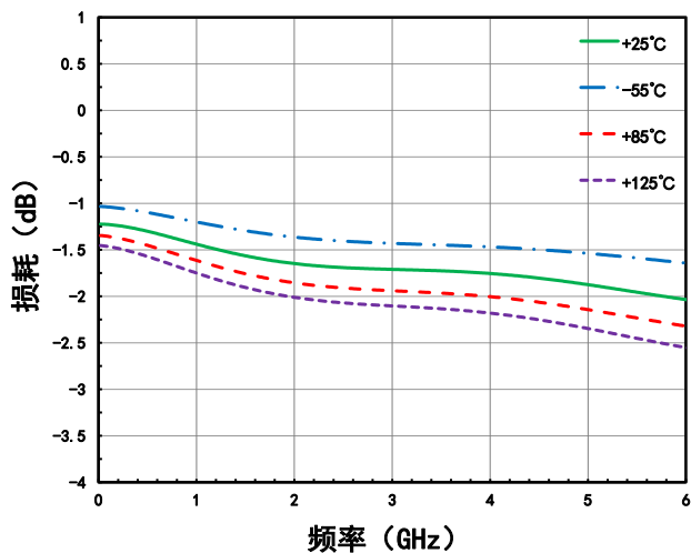
损耗 VS. 温度
