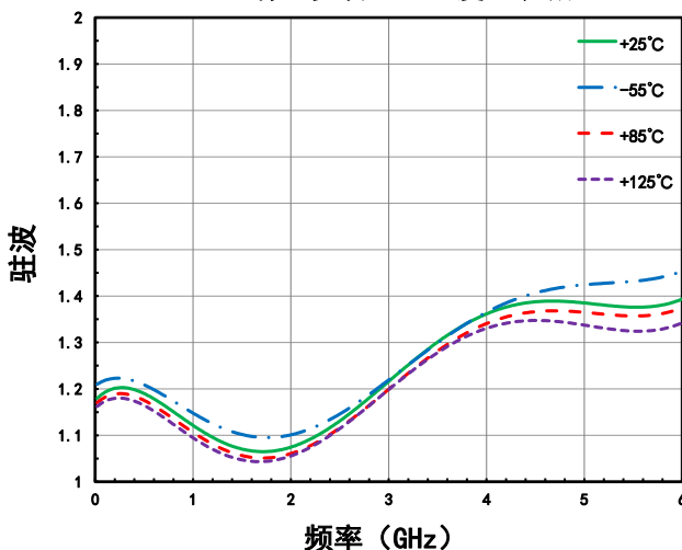
RF2端口驻波 VS. 温度 (衰减态)
