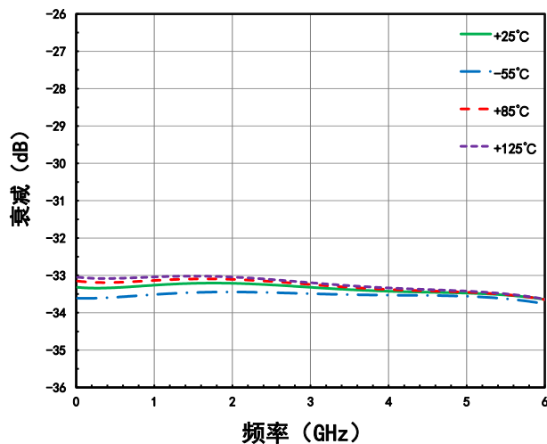
基本位衰减态 VS. 温度
