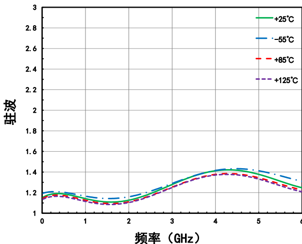
RF1端口驻波 VS. 温度 (衰减态)
