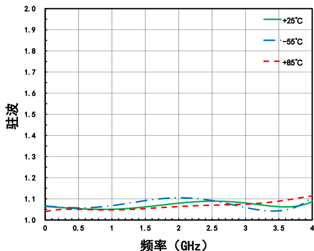
直通端驻波VS. 温度
