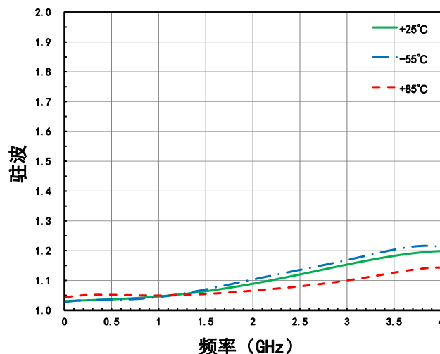
耦合端驻波VS. 温度
